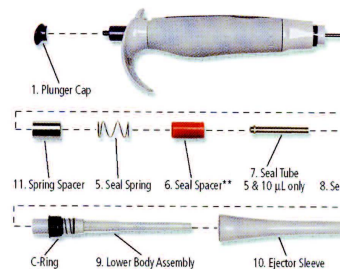
5 µL - 300 µL Pipettes
